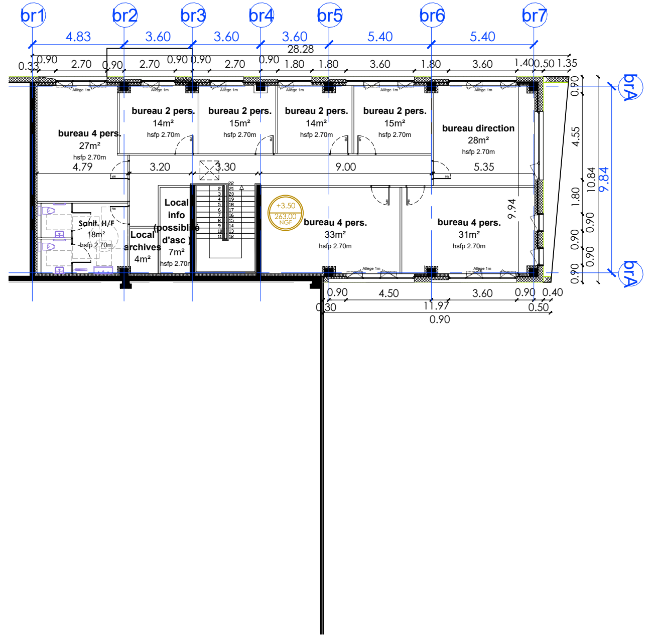
PLAN R+1 BUREAUX 1/200ème
